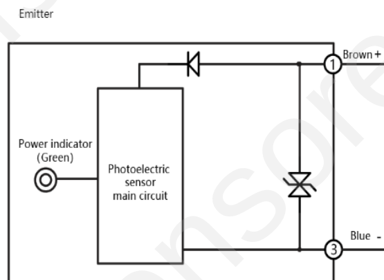
NPN
