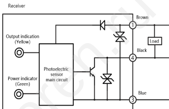
NPN
