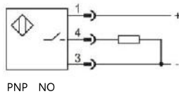
PNP NO
