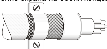
Заземление экрана на одном конце кабеля
