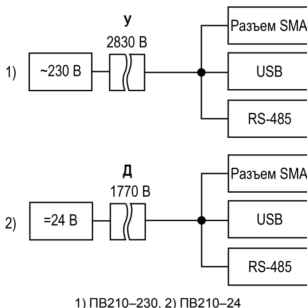
Рисунок 2.1 – Изоляция узлов прибора
