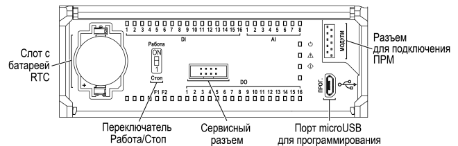
Рисунок 14 – Лицевая панель под крышкой
