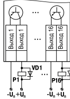
Рисунок 9 – Схема подключения нагрузок к ВЗ типа «К»
