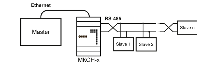
Рисунок 4 – Использование шлюза с подчиненными устройствами в интерфейсе RS-485
