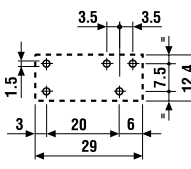
Вид сбоку
