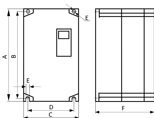
Рисунок 1 1,5...22 кВт (002Н...030Н)
