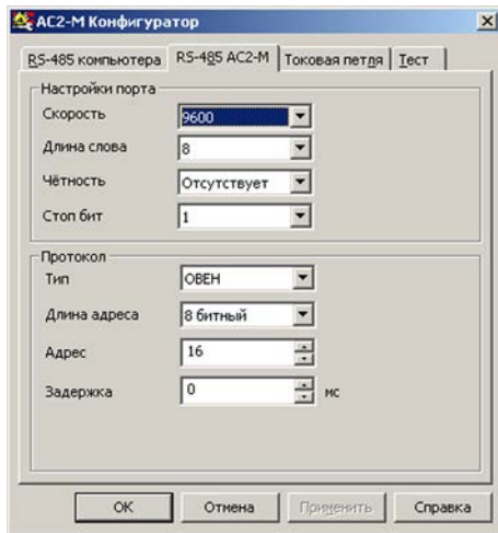
Рисунок 9.3 – Конфигуратор AC2-M. Вкладка «RS-485 AC2-M»
