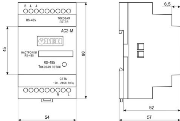
Рисунок А.1 - Габаритный чертеж преобразователя AC2-M
