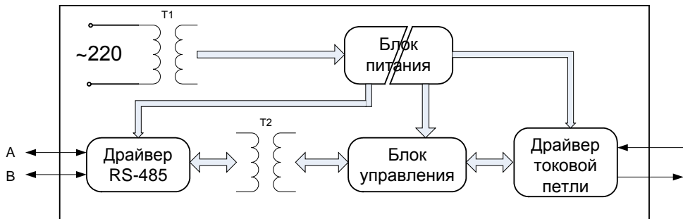
Рисунок 4.2 - Функциональная схема преобразователя
