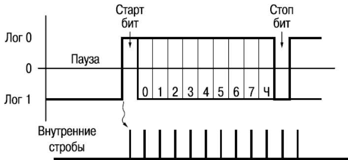
Рисунок 1.2 - Формат кадра передачи данных
