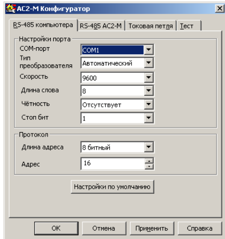
Рисунок 9.1 – Конфигуратор AC2-M. Вкладка «RS-485»
