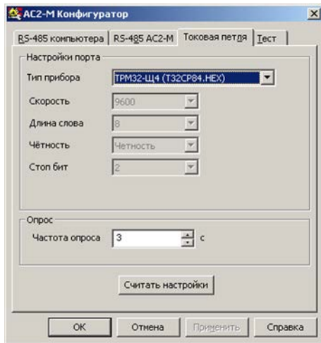
Рисунок 9.4 – Конфигуратор AC2-M. Вкладка «Токовая петля»
