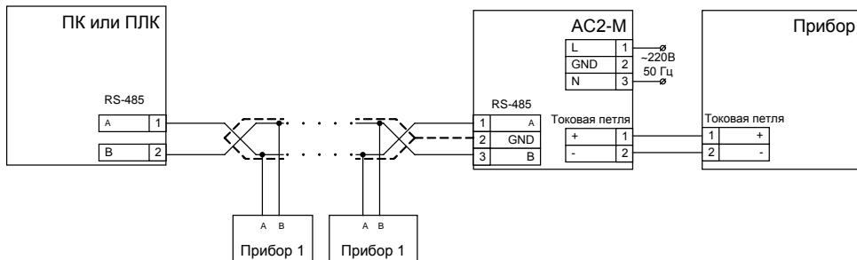
Рисунок 6.1 - Схема подключения преобразователя
