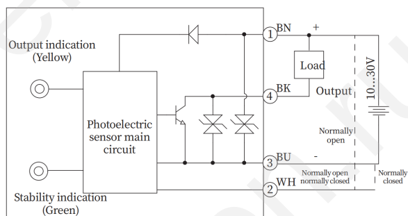
NPN
