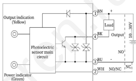
NPN
