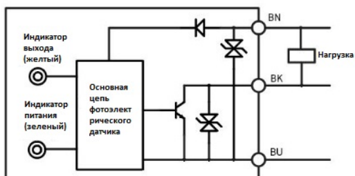
Приемник-NPN
