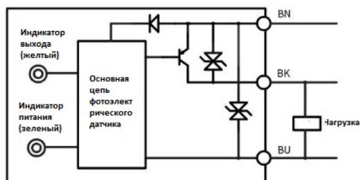
Приемник-PNP
